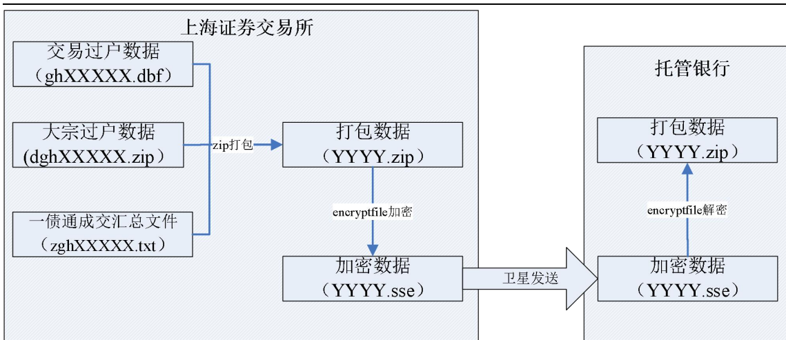
图 2 托管银行私有数据流图
